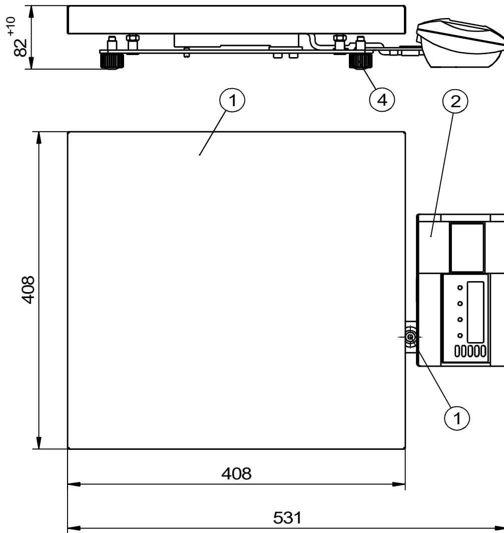
Rys.1. Wagi: TP-15/1, TP-30/1, TP-60/1 1- pomost, 2-miernik, 3-poziomniczka, 4-nóżka
