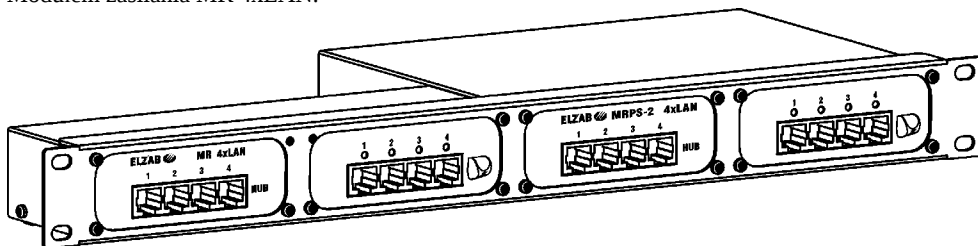
Rys. 7. Przykład rozbudowanego Modułu Zasilania MRPS-2 4xLAN + MR 4xLAN
